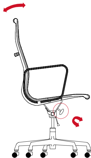
REGULACIÓN DE TENSIÓN DE BASCULACIÓN
